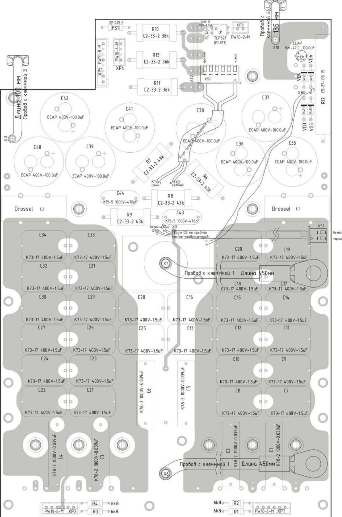
ВД-253, ВД-315 СБ Плата инвертора NB-IGBT-380 (1215)
