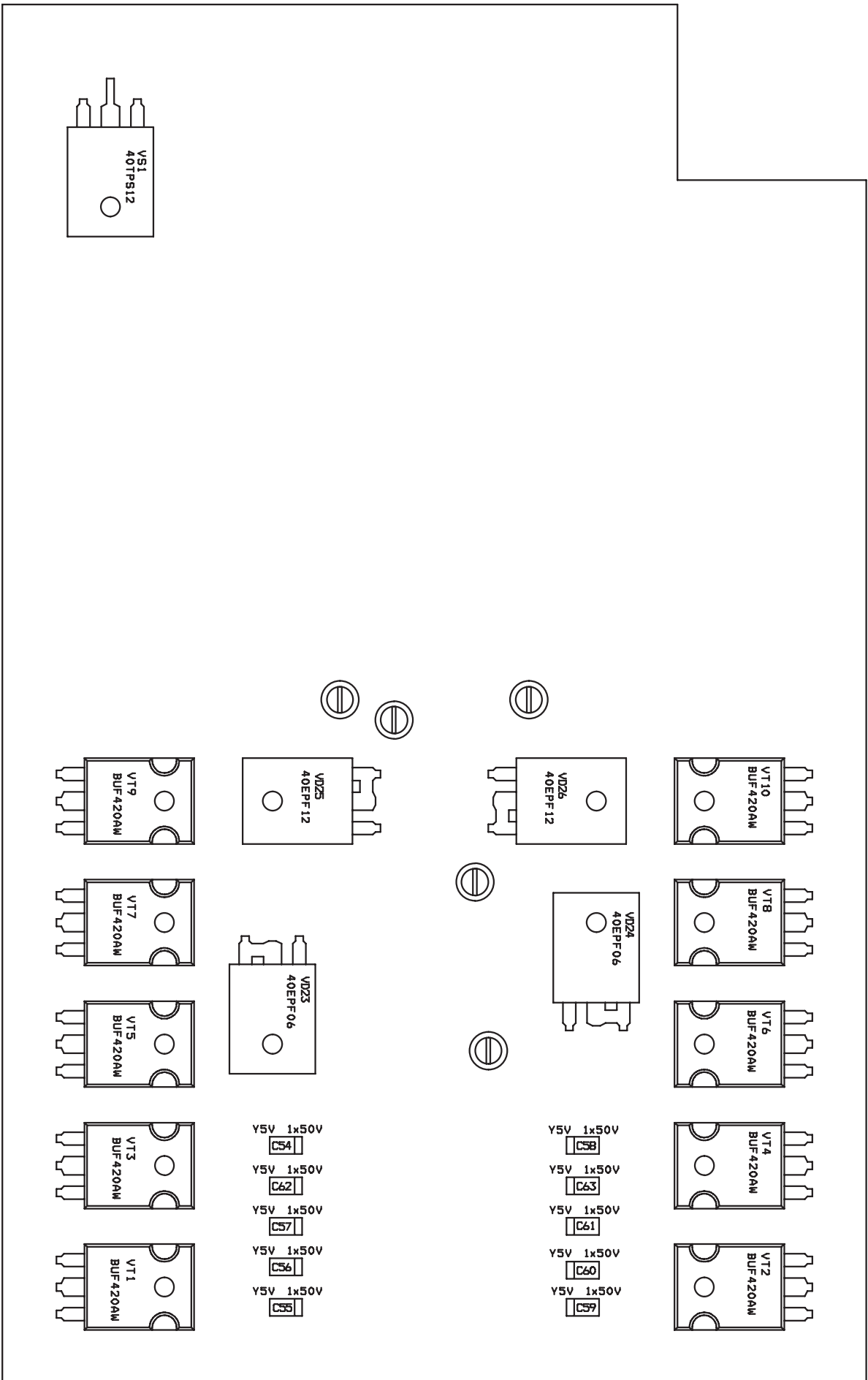
ВД-315 01.2000 СБ Плата инвертора
