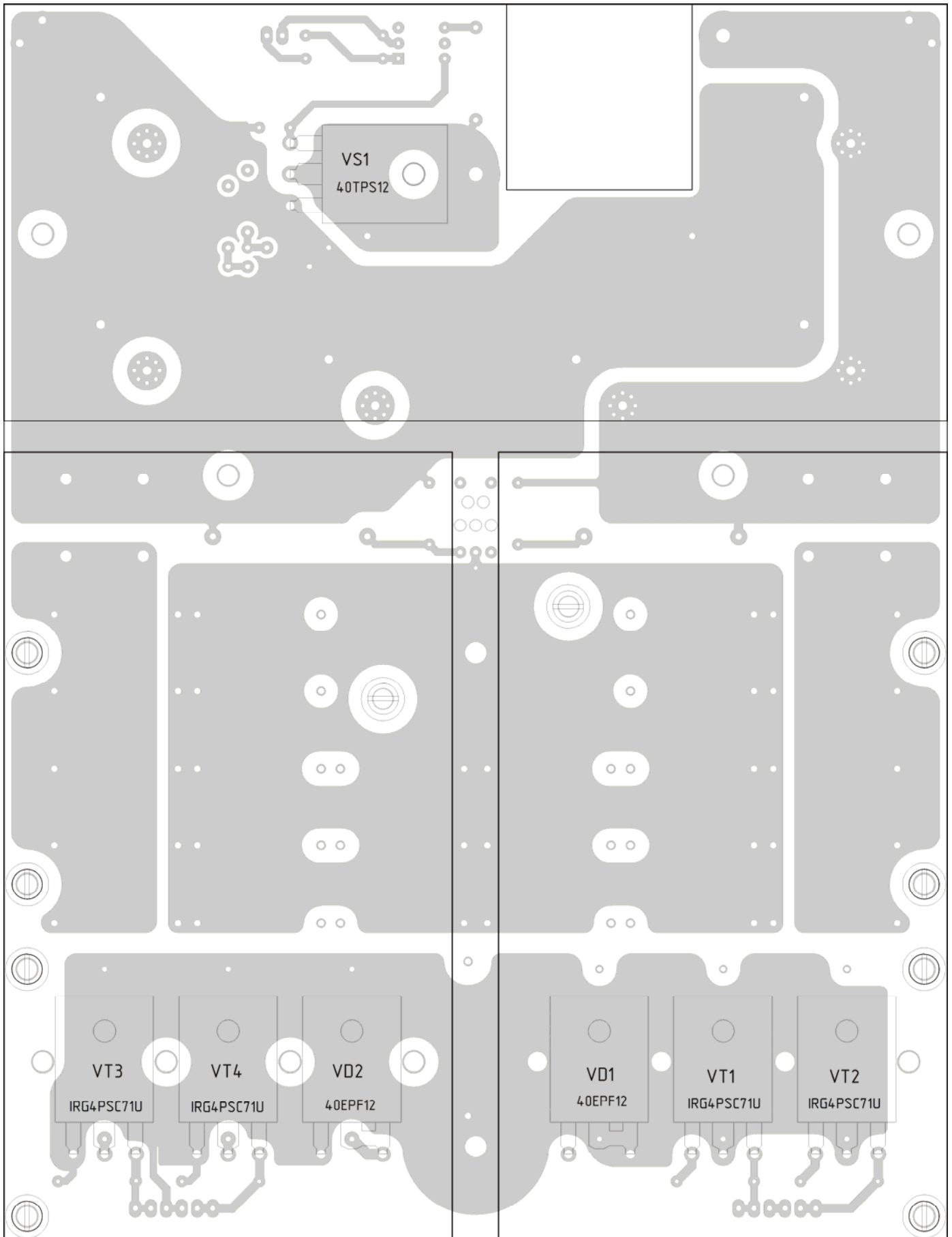
ВД-201 СБ Плата инвертора HB-IGBT-201 (1145)
