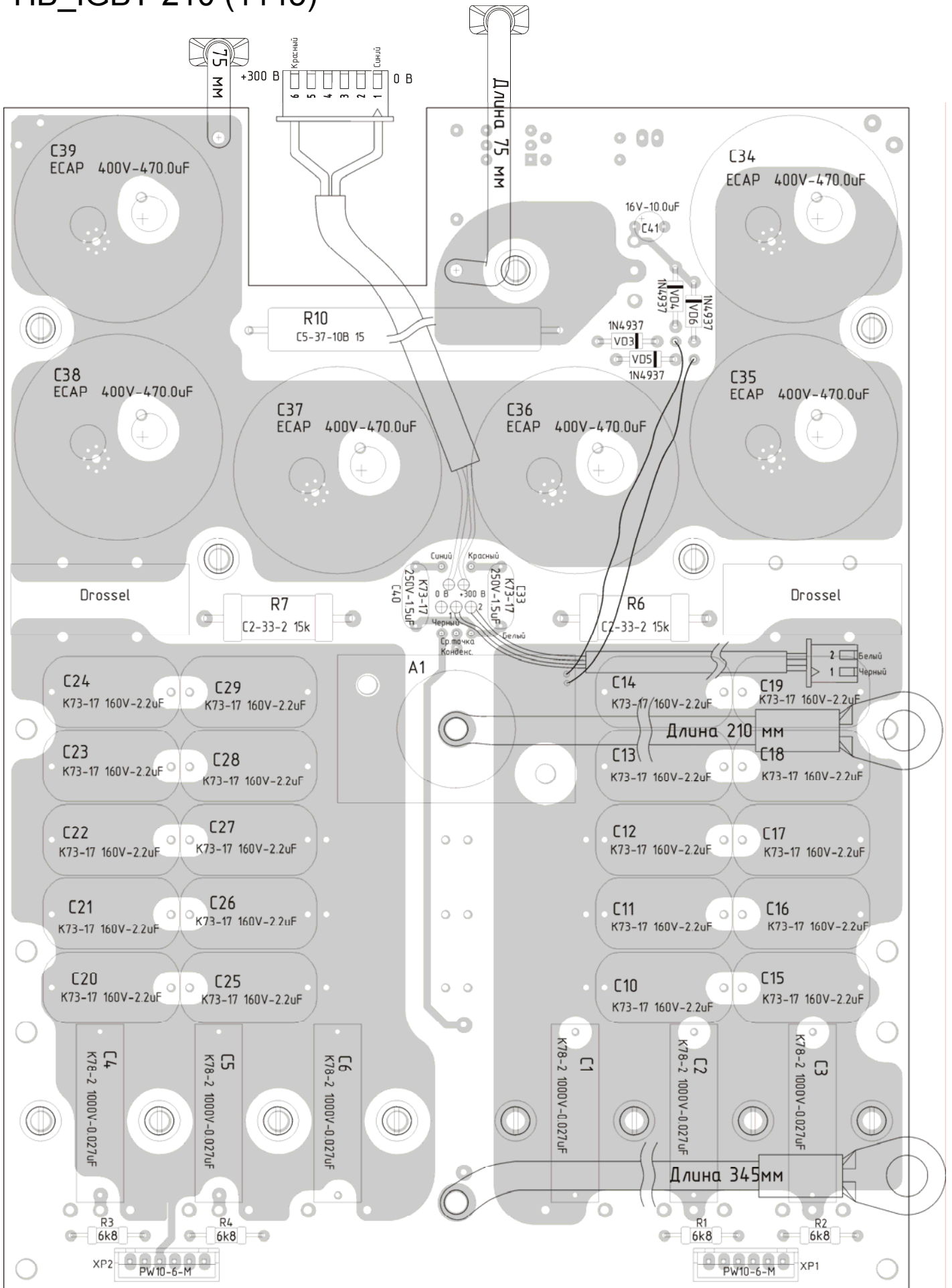
ВД-201 СБ Плата инвертора HB-IGBT-201 (1145)
