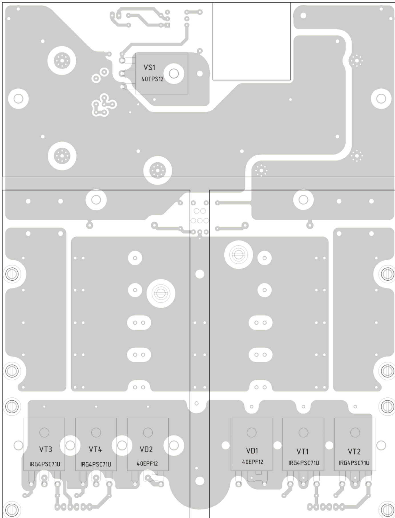
ВД-201 СБ Плата инвертора HB-IGBT-201 (1145)
