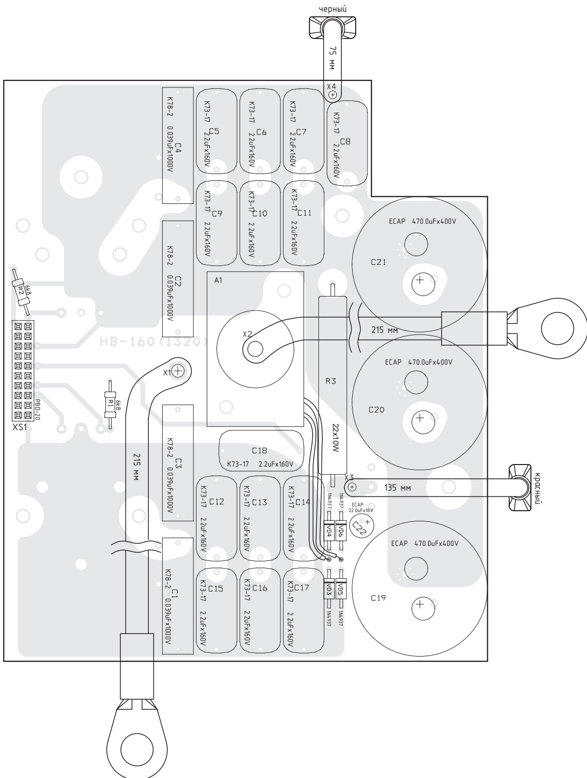
ЭИ.010.020 Инвертор ВД-160 НВ-160(1320)
