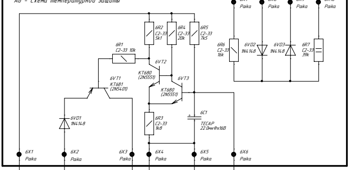
A6 - Схема температурной защиты
